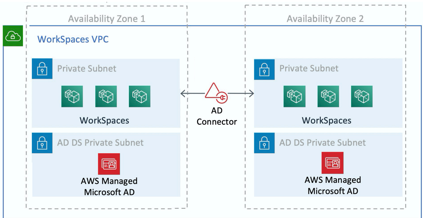
Abbildung 13: AD-DS-Netzwerkstruktur
