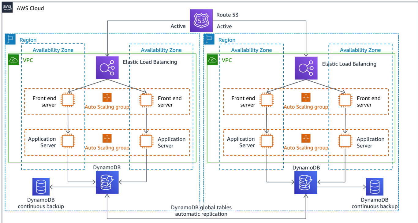
Abbildung 12: active/active Architektur mit mehreren Standorten (ändern Sie einen aktiven Pfad in Inaktiv für Hot-Standby)
