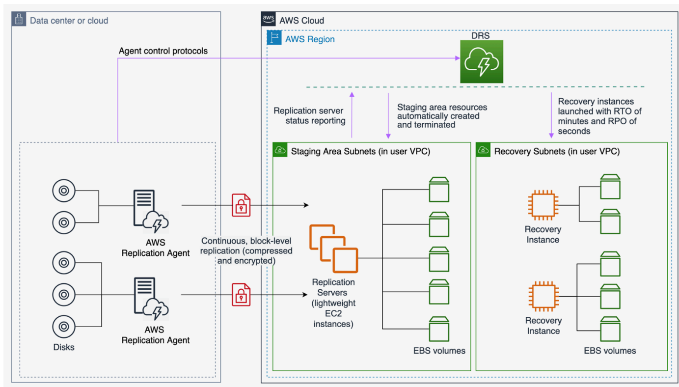
図 10 - AWS Elastic Disaster Recovery アーキテクチャ
