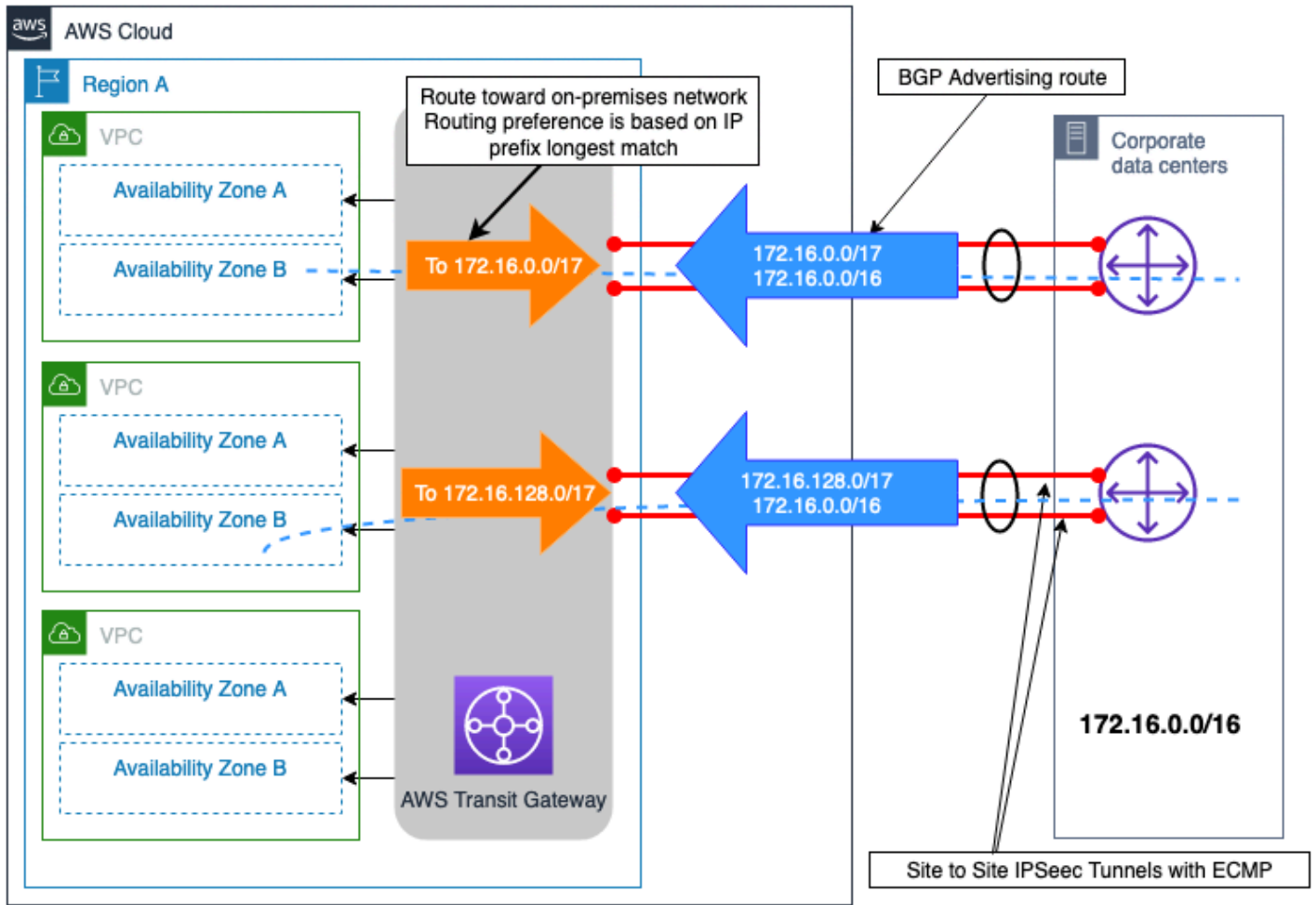
그림 10 - 더 구체적인 경로를 사용한 이중 Site-to-Site VPN 연결 예제
