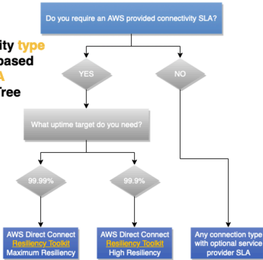
그림 3 - SLA 고려 결정 트리
