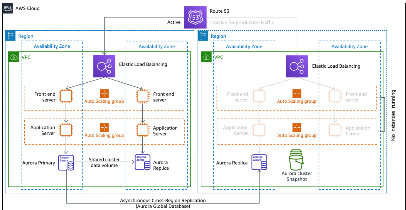
Figura 9: Arquitetura da luz piloto
