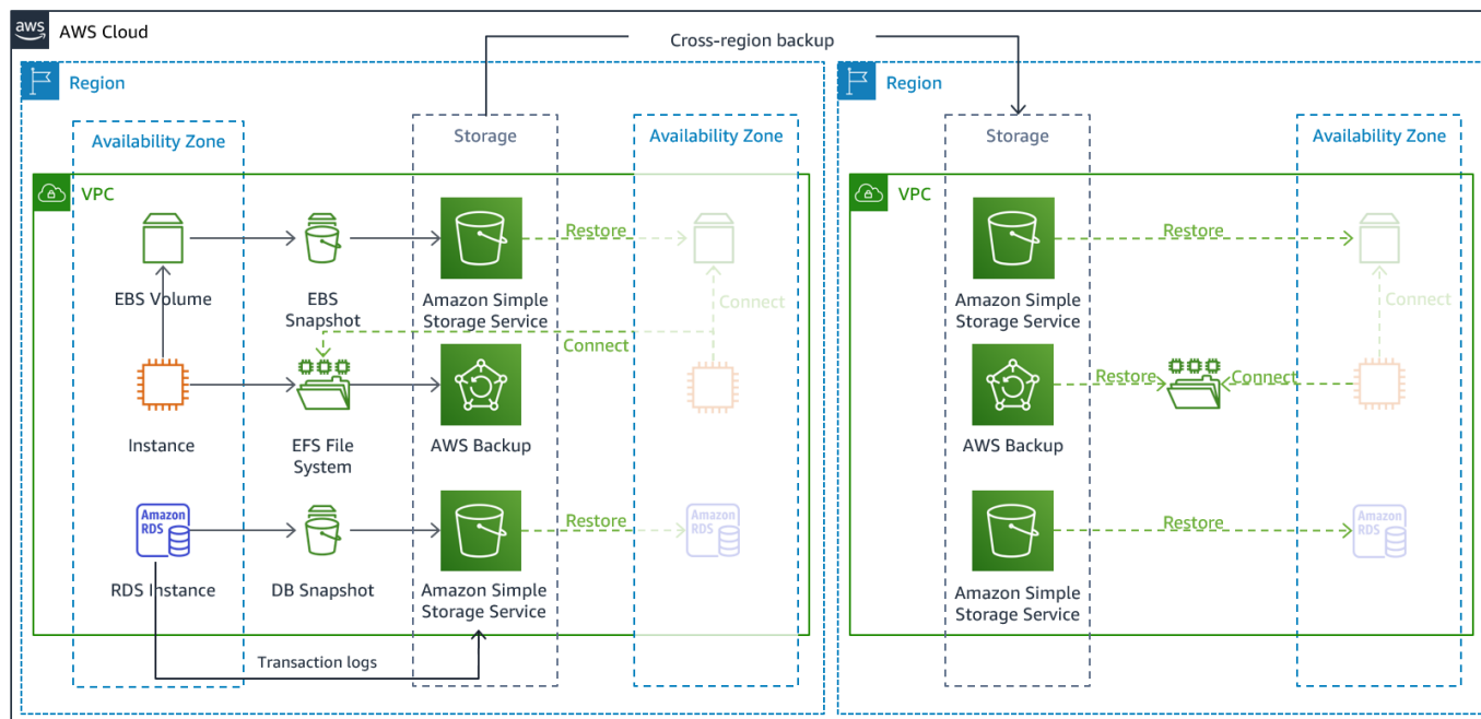
图 7-Backup 和恢复架构
